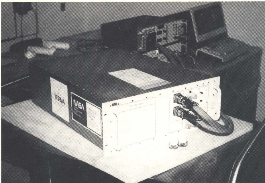
Denne metalæske er det danske Spacelab-1 eksperiment, en ovn til krystaldyrkningsforsøg. Ovnene er bygget af TERMA Elektronik A/S i Lystrup. I baggrunden ses et computeranlæg, som er ved at hente måledata ud fra ovnen, endnu inden den er åbnet efter flyvningen. Foto: OJK
